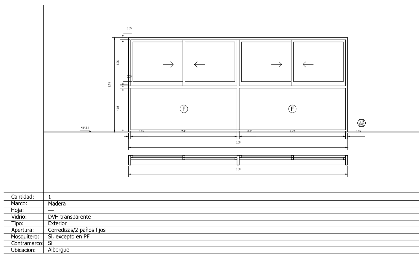
PLANILLA CARPINTERÍAS.Esc. 1:50. reducción de esc. 1:25
